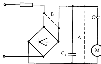
串联电路
